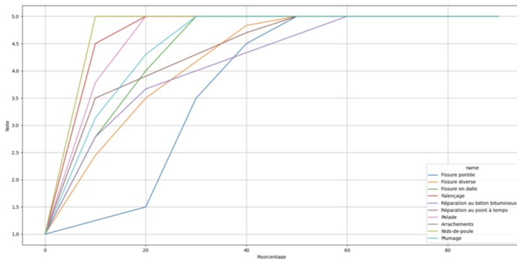
^ Diagramme des dégradations principales pour l'évaluation de la voirie.
