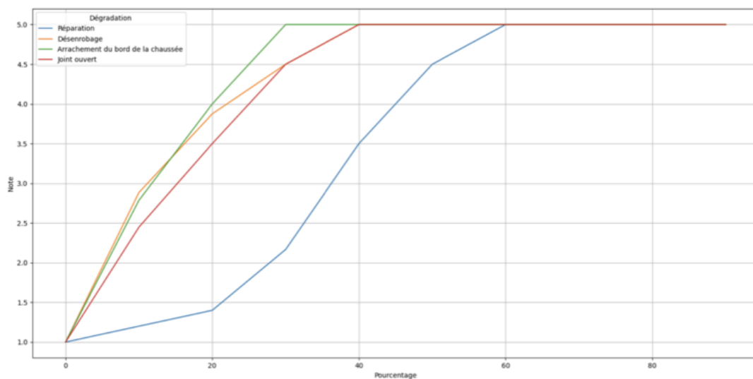
^ Diagramme des dégradations secondaires pour l'évaluation de la voirie.
